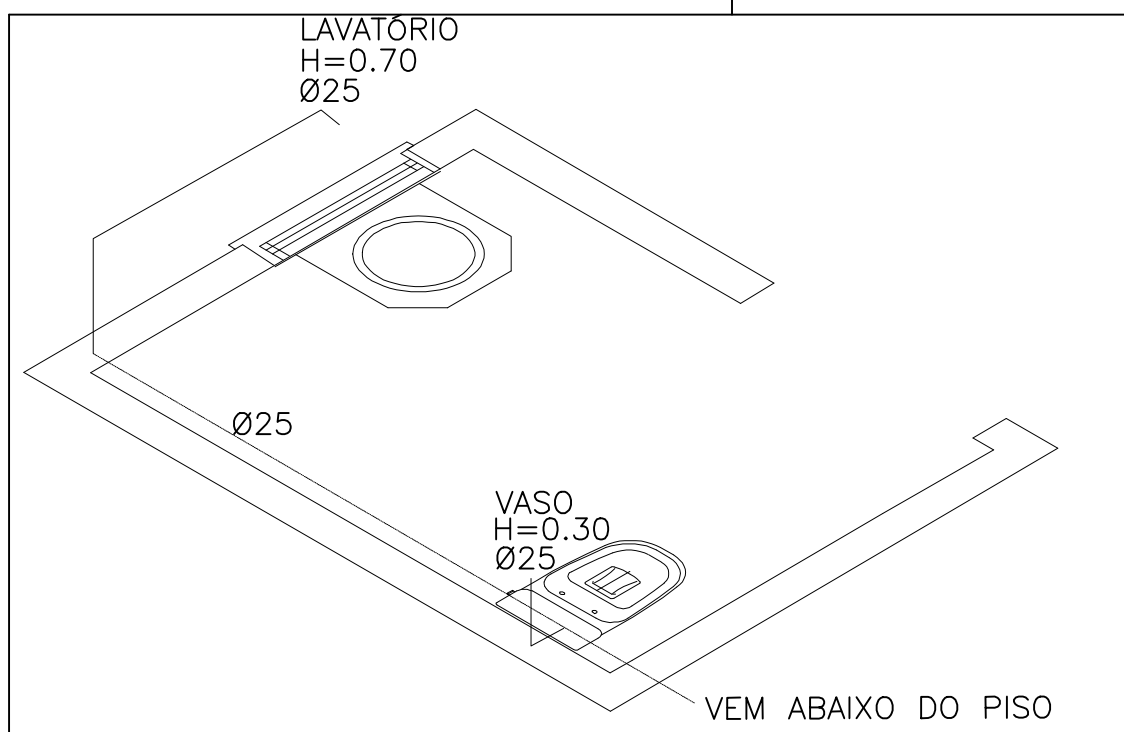
ISOMÉTRICO BANHEIRO FEM. SEM ESCALA SUMIDOURO
