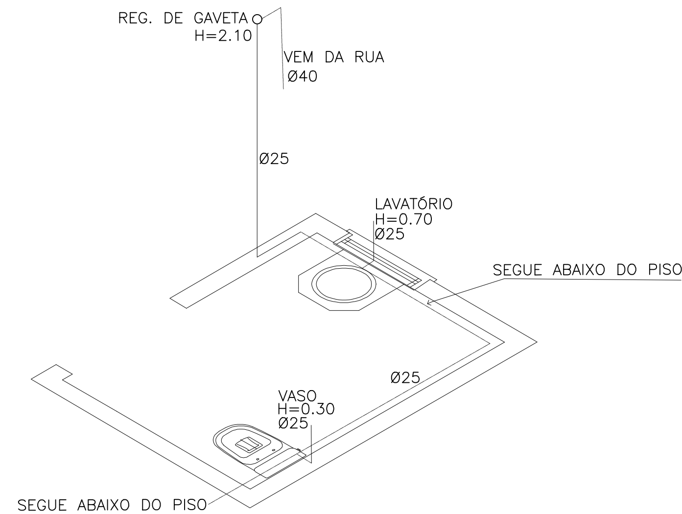
ISOMÉTRICO BANHEIRO MASC. SEM ESCALA
